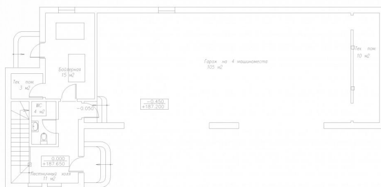
План 1 этажа
