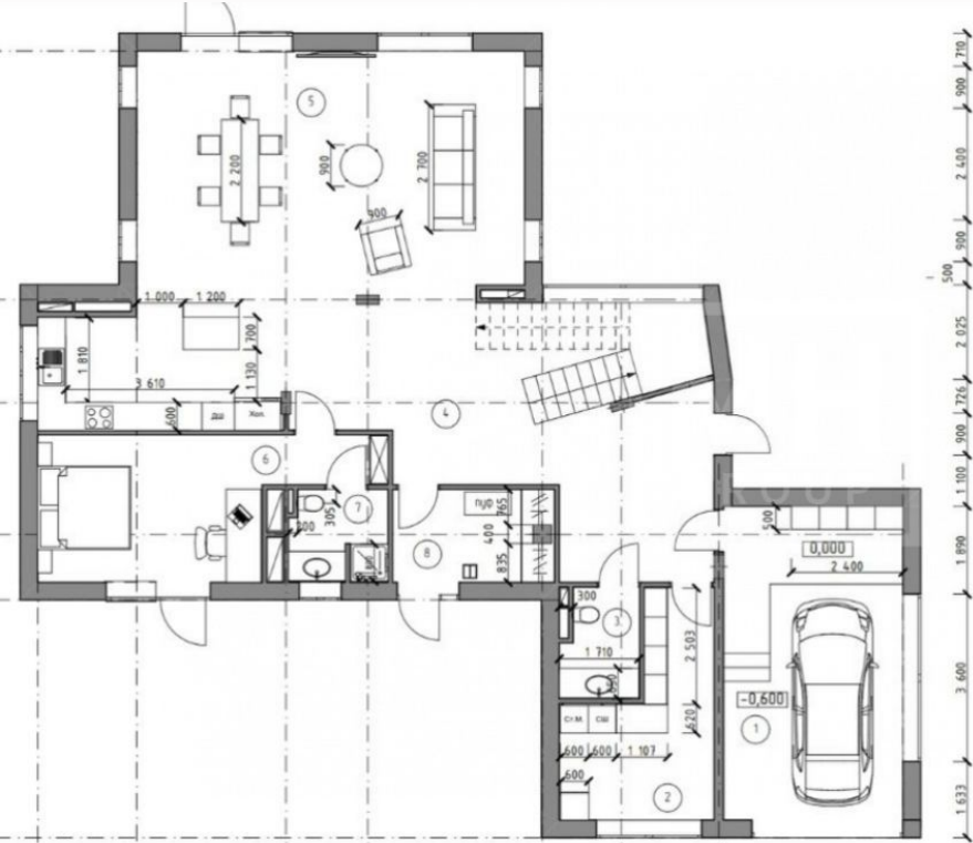
Экспликация помещений 1 этажа после перепланировки
